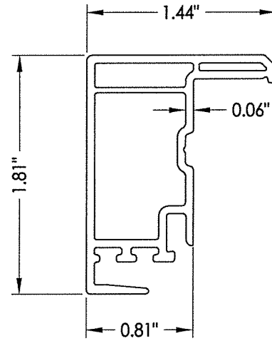
7 LOCK STILE
