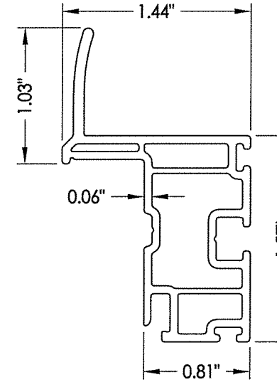
8 HANDLE STILE
